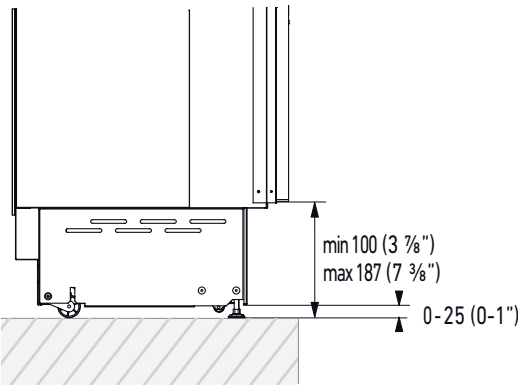
PLINTH SIZE
