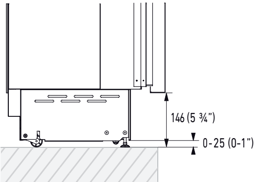
PLINTH SIZE
