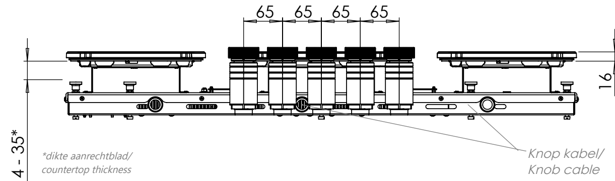
Vooraanzicht / Front view
