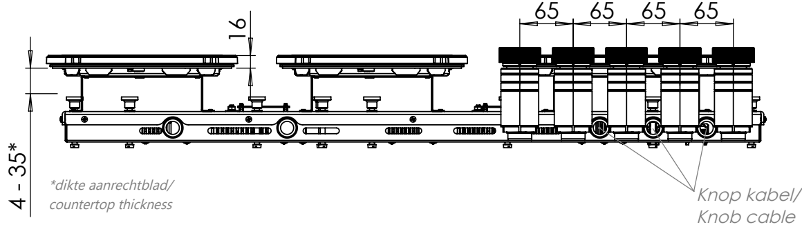
Vooraanzicht / Front view
