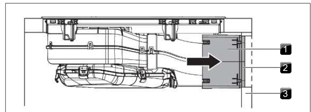
Afb. 9.20 Aansluiting op de achterwand
