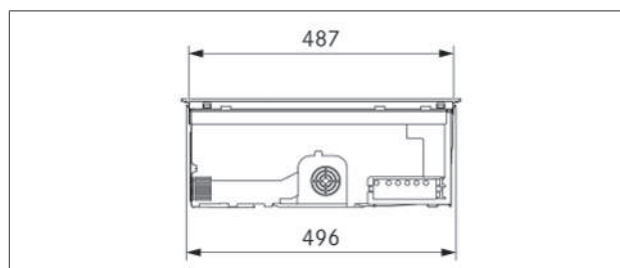
Afb. 3.3 Apparaatafmetingen zijaanzicht
