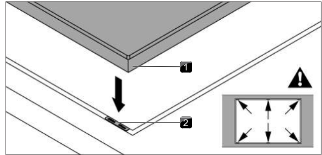
Afb. 9.18 Vulplaatjes invoegen
