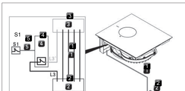
Afb. 9.27 Aansluitschema met externe schakelcontacten
