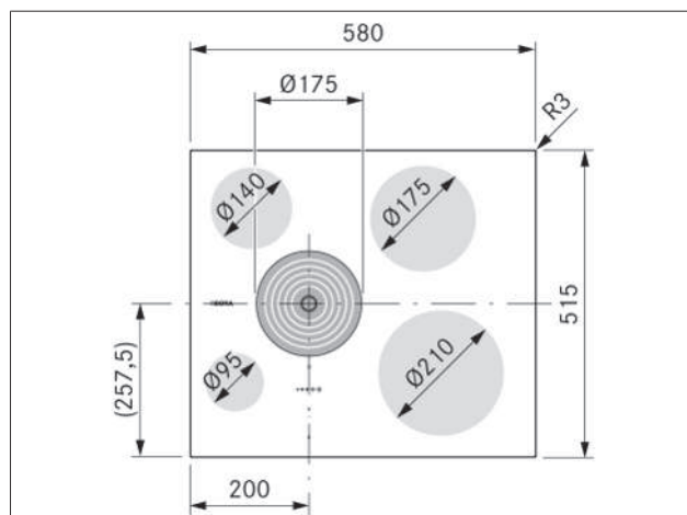
Afb. 3.1 Apparaatafmetingen bovenaanzicht
