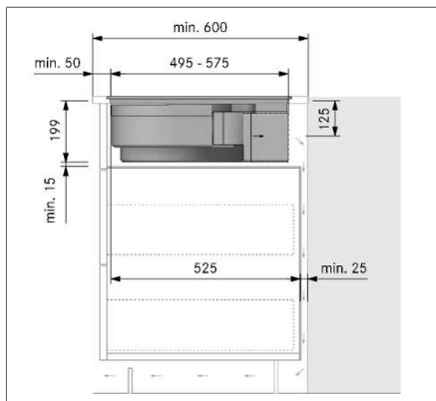
Afb. 9.13 Inbouwmaten bij recirculatie - montagevariant B, werkblad diepte 600 mm
