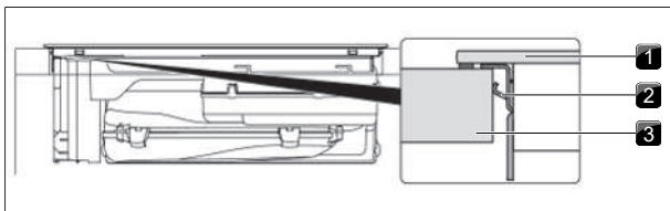
Afb. 9.17 Kookveld bevestigen
