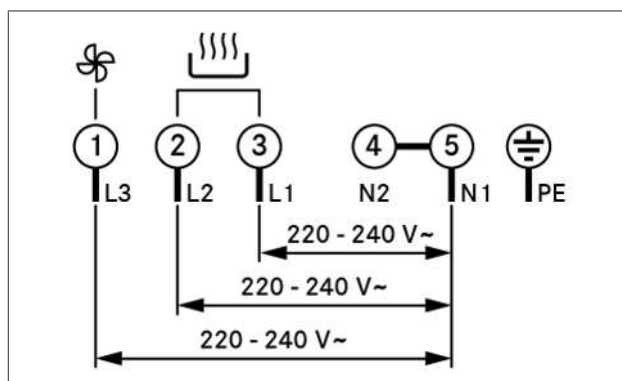
Afb. 9.23 Aansluitschema 3-fasig
