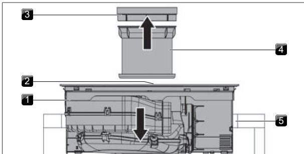
Afb. 9.16 Kookveld plaatsen
