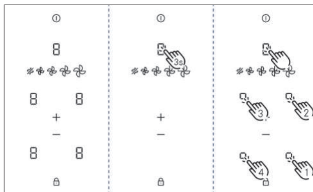
Afb. 9.28 Display dealer- en servicemenu oproepen
