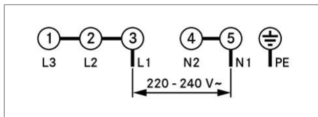
Afb. 9.25 Aansluitschema 1-fasig
