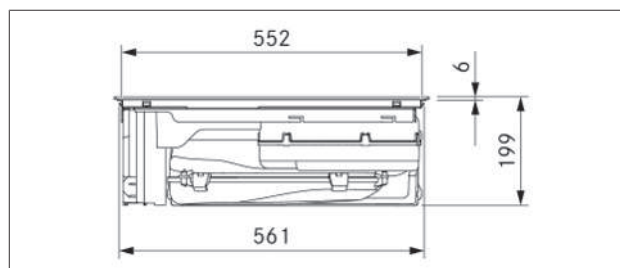
Afb. 3.2 Apparaatafmetingen vooraanzicht
