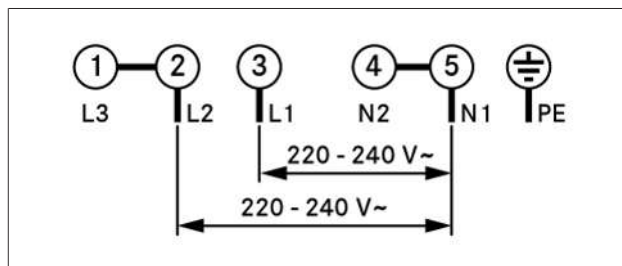
Afb. 9.24 Aansluitschema 2-fasig
