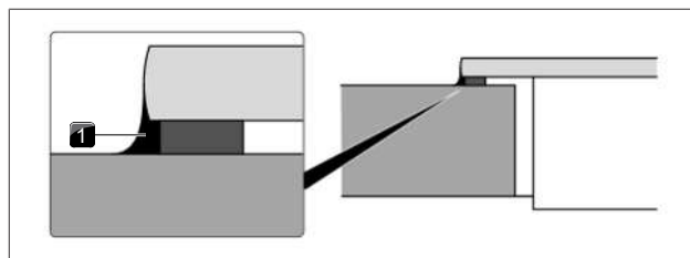
Afb. 9.31 Siliconenkit bij opbouwmontage
