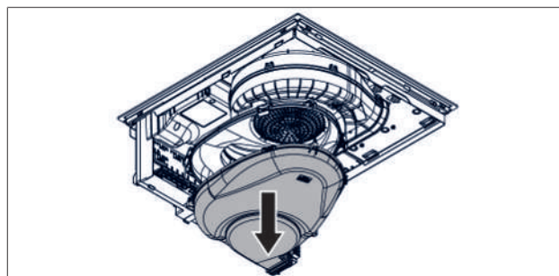
Afb. 9.22 Het onderste deel van de zuigkamer demonteren
