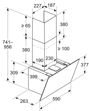
Afmeting in mm Apparaat in luchtafvoermodus
