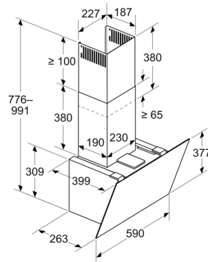
Afmeting in mm Apparaat in luchtcirculatiemodus
