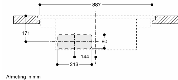
Vooraanzicht - Meubeluitsparing voor ongeleide circulatie - vlak (CA 082 010)
