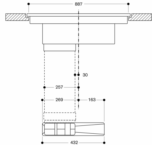
Frontaanzicht van CV 492 met kanaal-luchtrecirculatie
