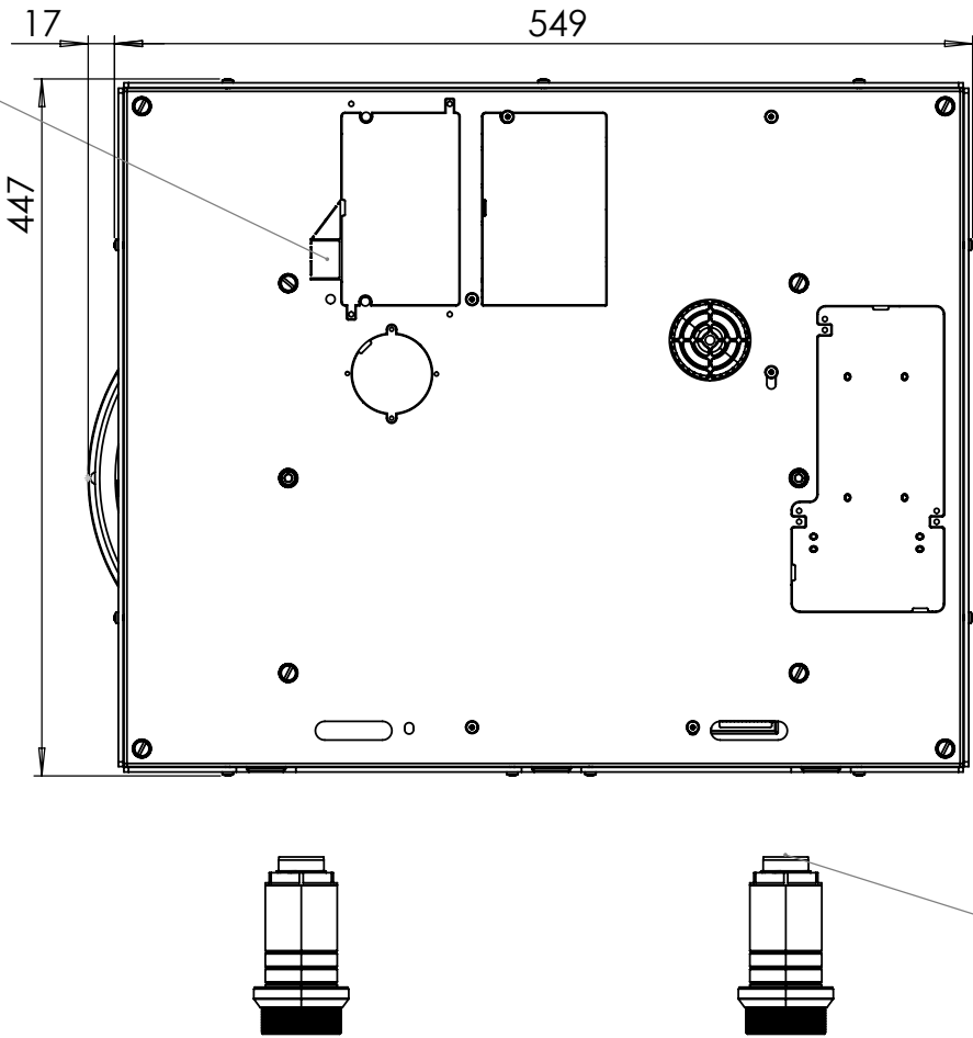
Onderaanzicht / Bottom view
