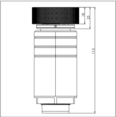
Vooraanzicht bedieningsknop
