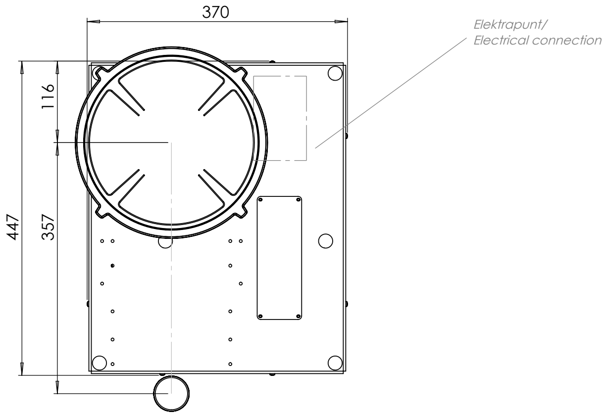
Bovenaanzicht / Top view
