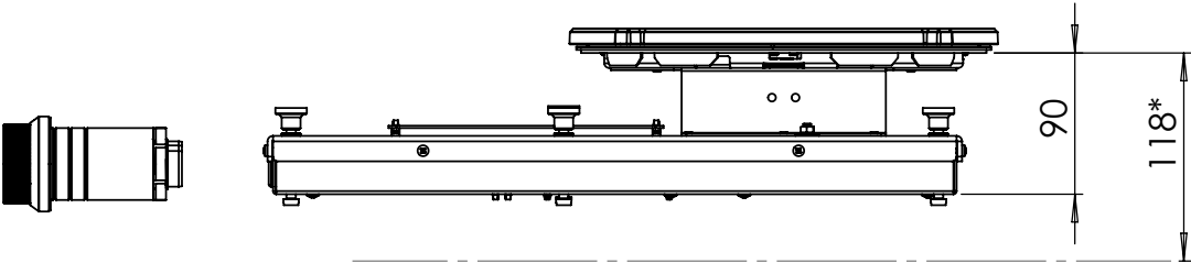
Zijaanzicht / Side view
