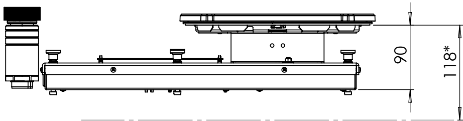
Zijaanzicht / Side view
