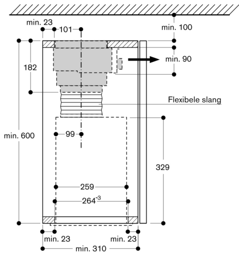
Dwarsdoorsnede bovenkast met AC 200 en AA 211 812
